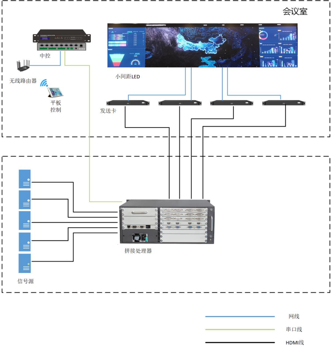
系统拓扑图
