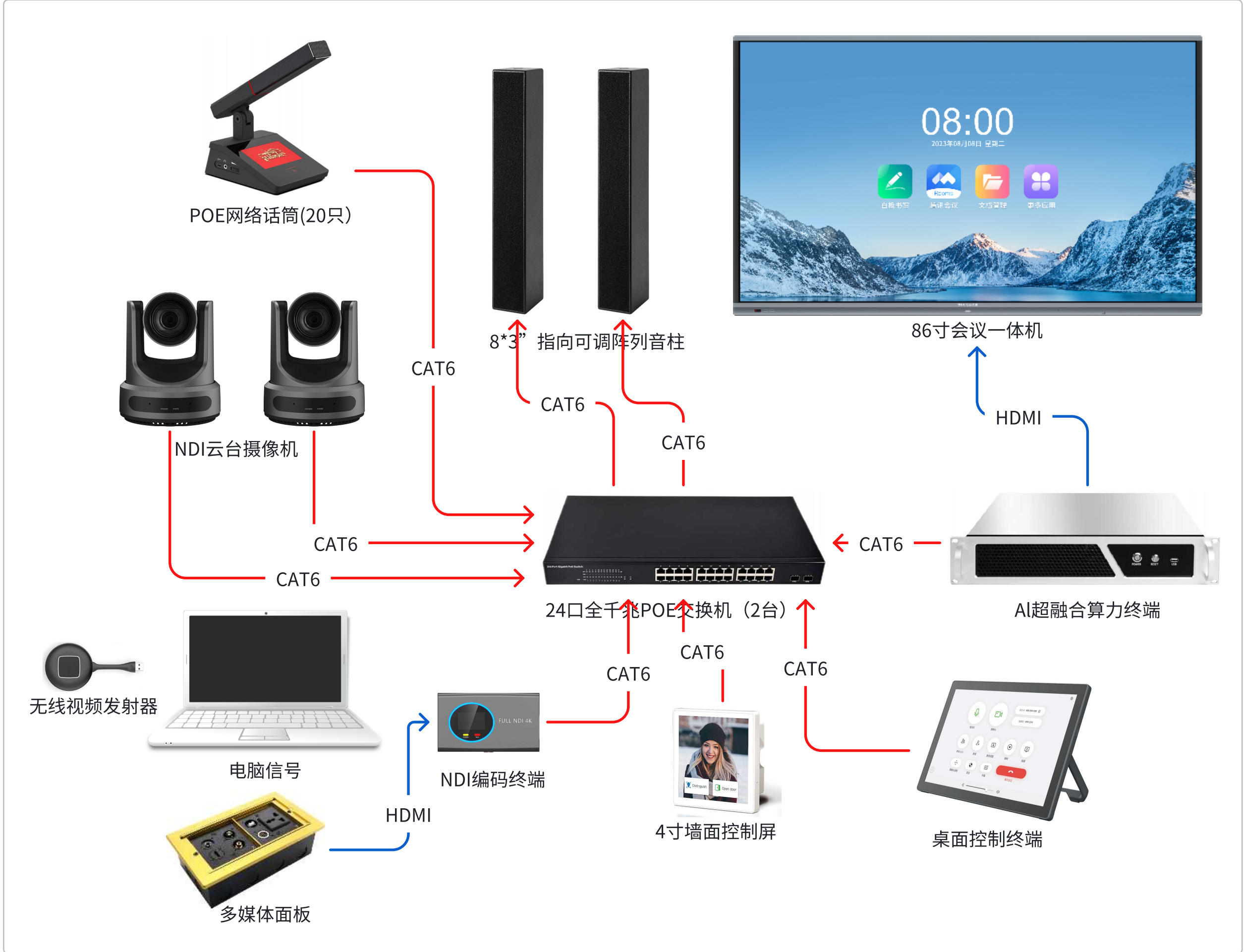
10-20人会议室系统架构图
