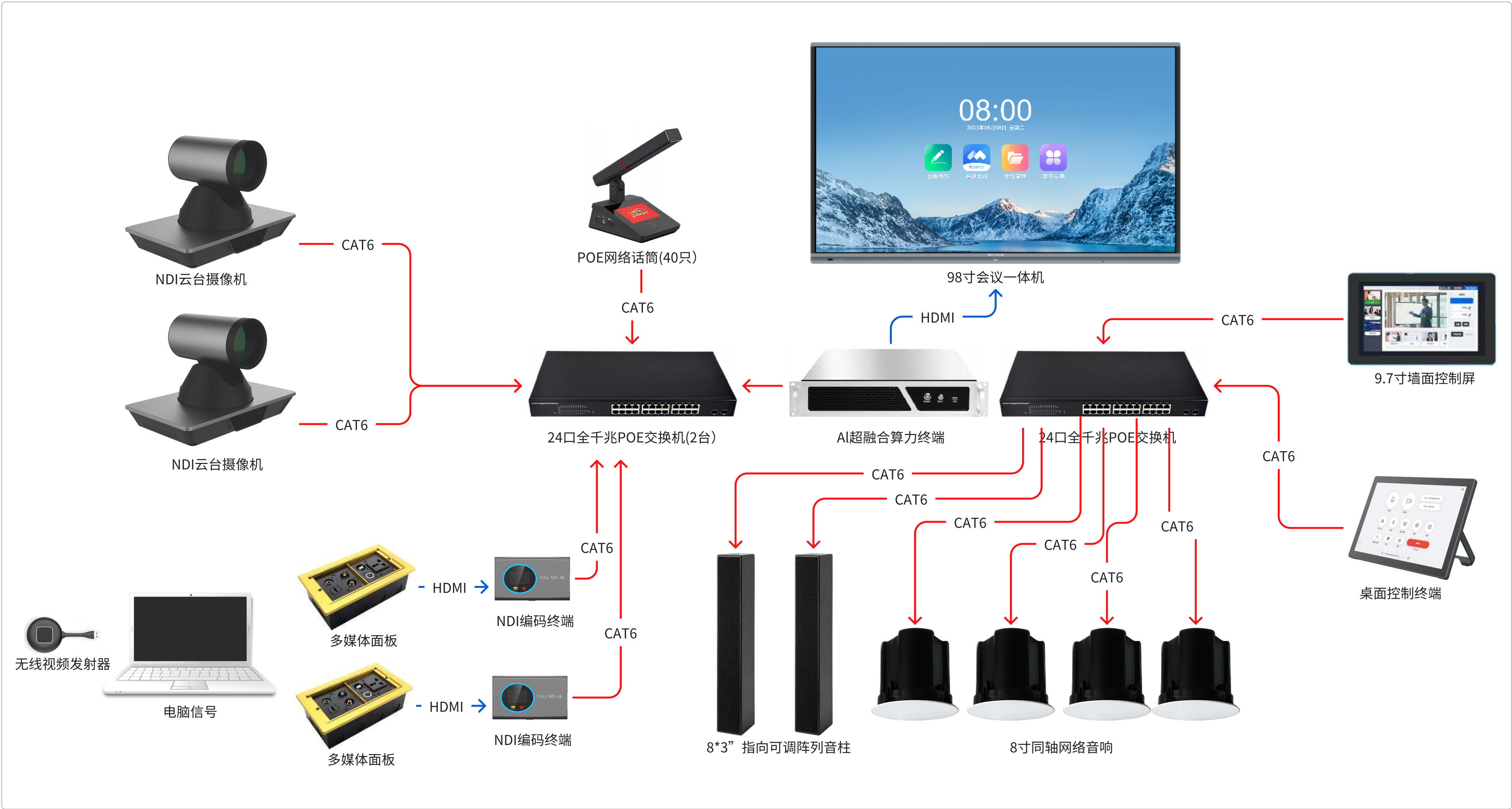
20-40人大会议室系统架构图
